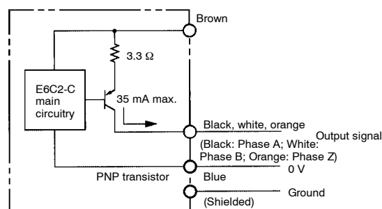
E6C2-CWZ5B
